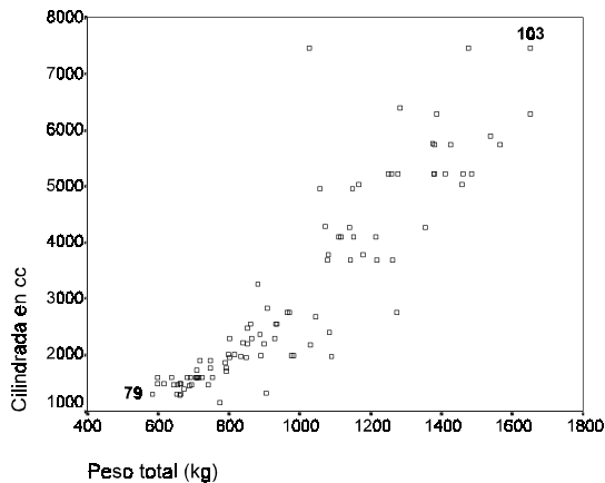
Figura 21.2. Diagrama de dispersión del peso por la cilindrada.
