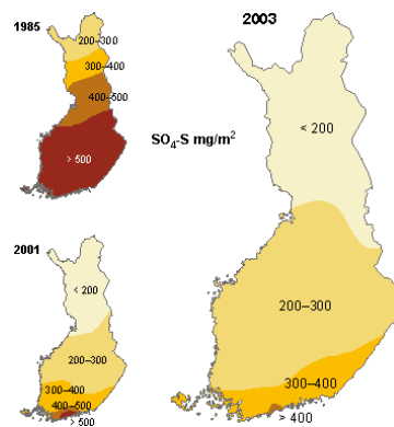
Veden happamuus Suomessa
